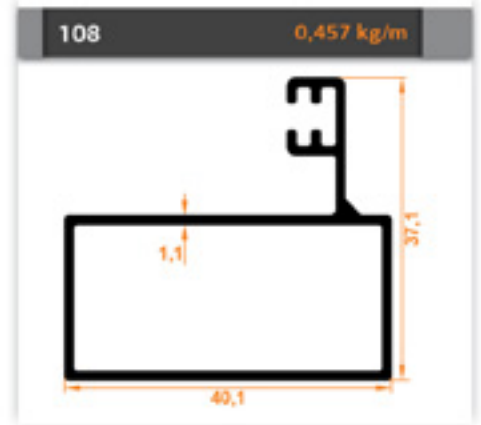
Geniş Yan Dikme Wide Side Column
