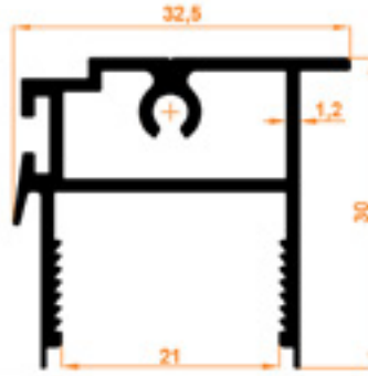
Çekme Baza Pull Base Profile
