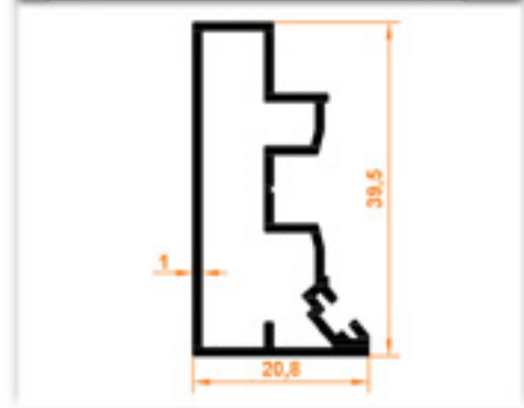
Yan Dikme Profili Side Column Profile
