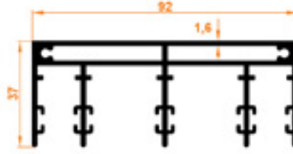
3'lü Üst Kasa Triple Top Case Profile
