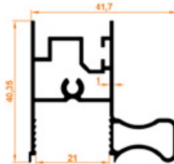
Sürme Birleştirme Kilit Karşılık Profili Sliding Combination Lock Provision Profile
