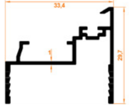
Sabit Cam Kilit Karşılığı Profili Constant Glass Lock Provision Profile
