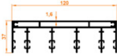
4'lü Üst Kasa Quadruple Top Case Profile
